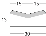
Cuneta R4
