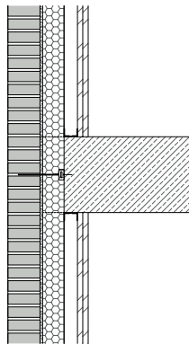
Secció Ferrater brick 12
