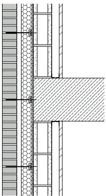
Secció Ferrater brick 9,5
